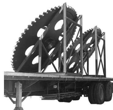
SPROCKET ACCU-TORCH® DE 3 M DE DIÁMETRO UTILIZADO EN FABRICAS DE PAPEL
